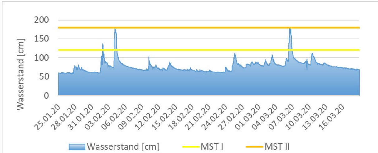
Abbildung 23: Wasserstand und Meldestufenüberschreitungen am Pegel Eberstadt / Modau 25. Januar bis 18. März 2020. Meldestufe 1 = 120cm (gelbe Linie), Meldestufe 2 = 180 cm (orangefarbene Linie), Meldestufe 3 = 230 cm (nicht in Grafik zu sehen)
