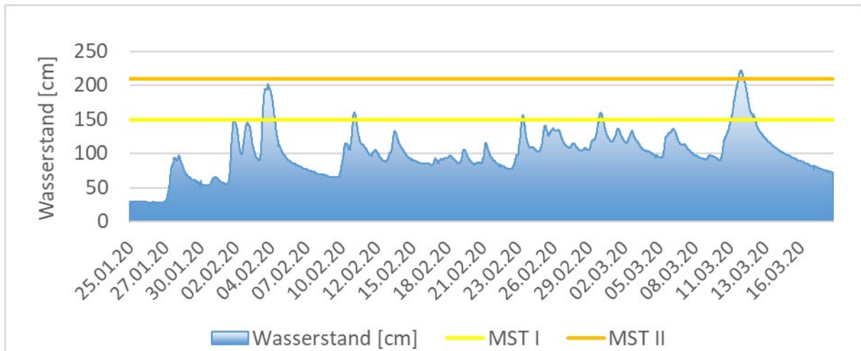
Abbildung 13: Wasserstand und Meldestufenüberschreitungen am Pegel Bronzell / Fulda 25. Januar bis 18. März 2020. Meldestufe 1 = 150 cm (gelbe Linie), Meldestufe 2 = 210 cm (orangefarbene Linie), Meldestufe 3 = 270 cm (nicht in Grafik zu sehen)
