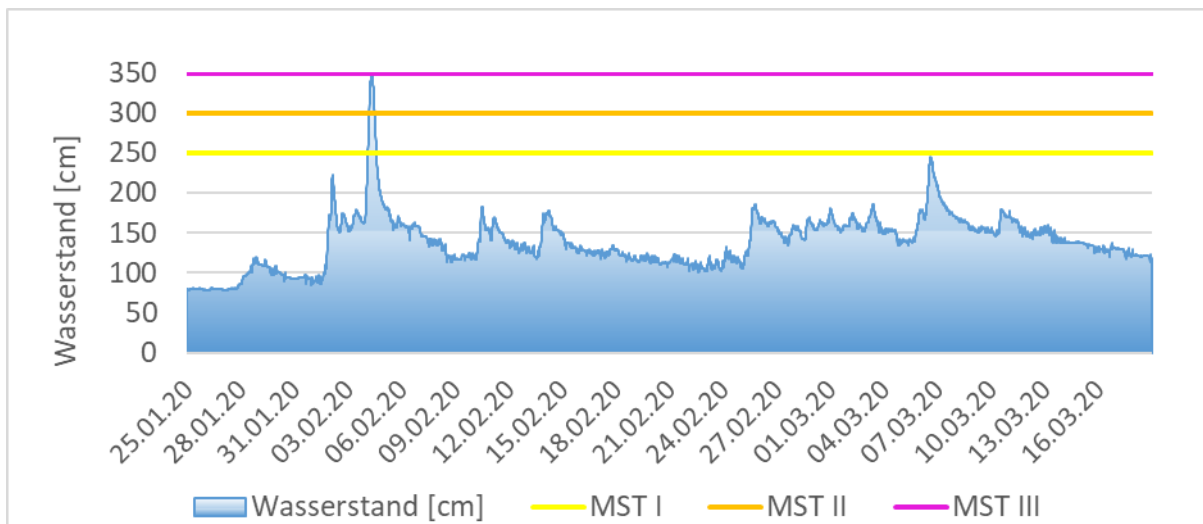
Abbildung 18: Wasserstand und Meldestufenüberschreitungen am Pegel Hainstadt / Mümling 25. Januar bis 18. März 2020. Meldestufe 1 = 250 cm (gelbe Linie), Meldestufe 2 = 300 cm (orangefarbene Linie), Meldestufe 3 = 350 cm (pinke Linie)
