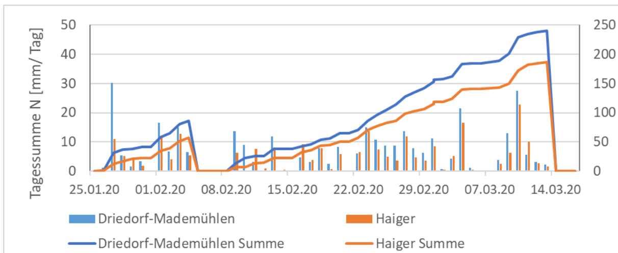
Abbildung 3: Tagesniederschlagssummen im Westerwald
