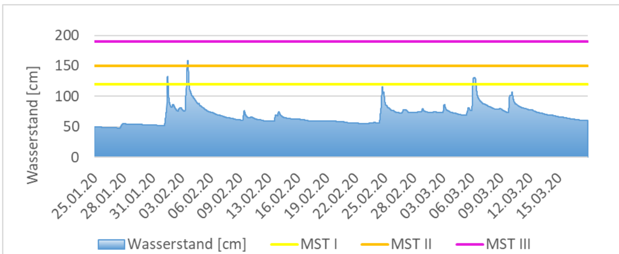
Abbildung 22: Wasserstand und Meldestufenüberschreitungen am Pegel Fahrenbach / Weschnitz 25. Januar bis 18. März 2020. Meldestufe 1 = 120 cm (gelbe Linie), Meldestufe 2 = 150 cm (orangefarbene Linie), Meldestufe 3 = 190 cm (pinke Linie)
