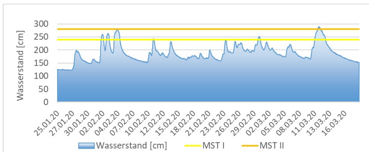
Abbildung 12: Wasserstand und Meldestufenüberschreitungen am Pegel Kerzell / Fliede 25. Januar bis 18. März 2020. Meldestufe 1 = 240 cm (gelbe Linie), Meldestufe 2 = 280 cm (orangefarbene Linie), Meldestufe 3 = 310 cm (nicht in Grafik zu sehen)
