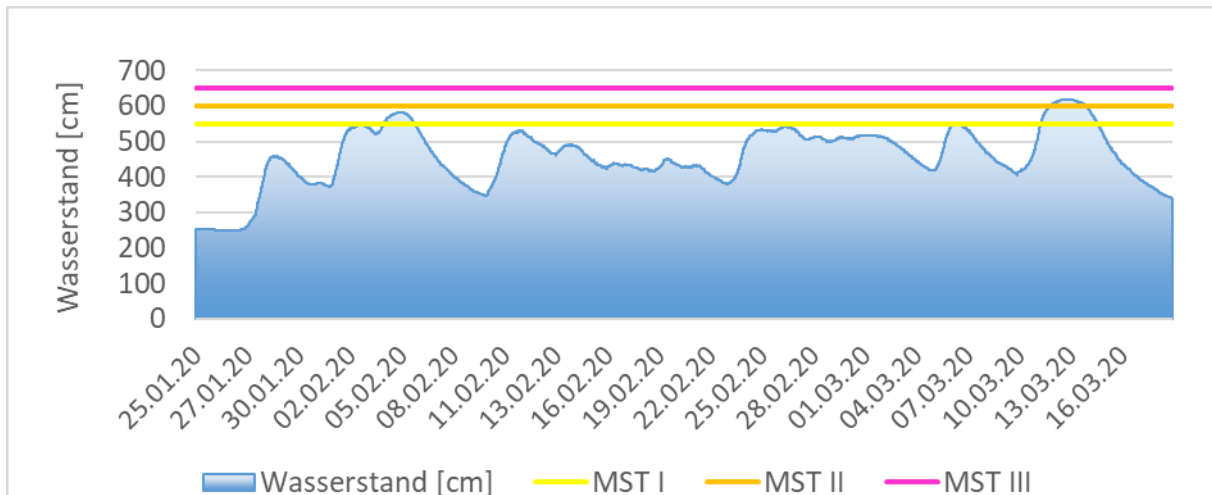
Abbildung 11: Wasserstand und Meldestufenüberschreitungen am Pegel Gießen / Lahn 25. Januar bis 18. März 2020. Meldestufe 1 = 550 cm (gelbe Linie), Meldestufe 2 = 600 cm (orangefarbene Linie), Meldestufe 3 = 650 cm (pinke Linie)
