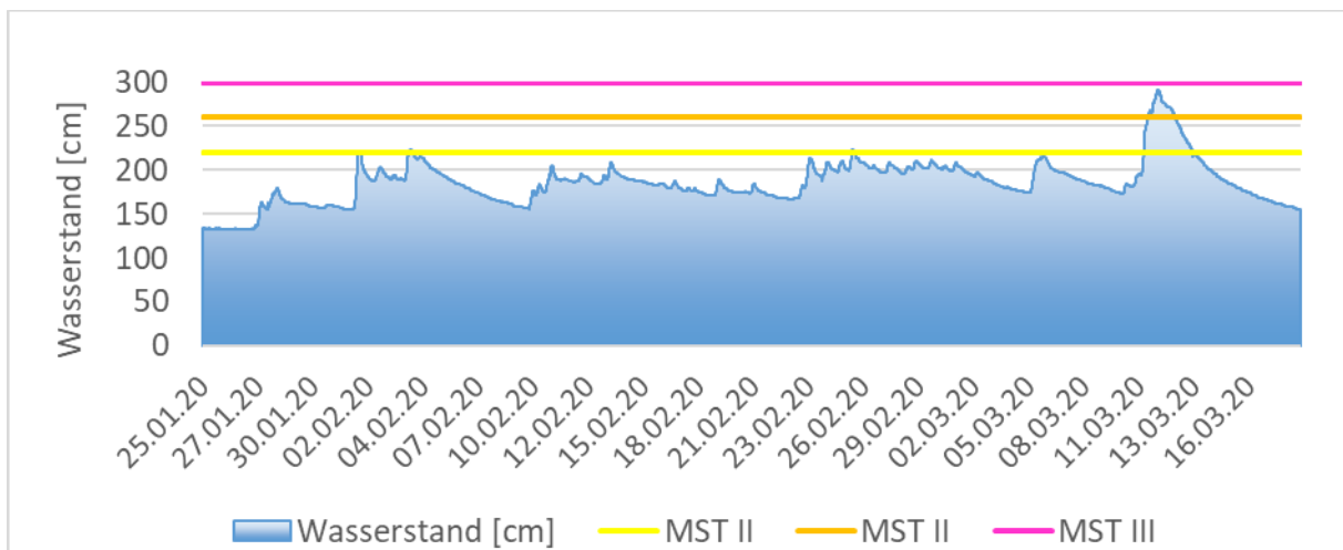
Abbildung 10: Wasserstand und Meldestufenüberschreitungen am Pegel Etzelmühle / Salzböde 25. Januar bis 18. März 2020. Meldestufe 1 = 220 cm (gelbe Linie), Meldestufe 2 = 260 cm (orangefarbene Linie), Meldestufe 3 = 300 cm (pinke Linie)
