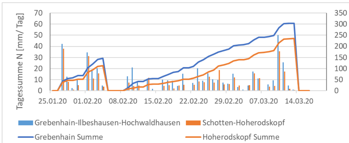
Abbildung 2: Tagesniederschlagssummen im Vogelsberg
