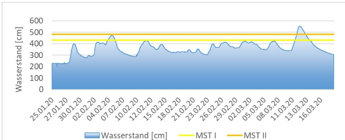
Abbildung 14: Wasserstand und Meldestufenüberschreitungen am Pegel Bad Hersfeld 1 / Fulda 25. Januar bis 18. März 2020. Meldestufe 1 = 430cm (gelbe Linie), Meldestufe 2 = 480 cm (orangefarbene Linie), Meldestufe 3 = 600 cm (nicht in Grafik zu sehen)
