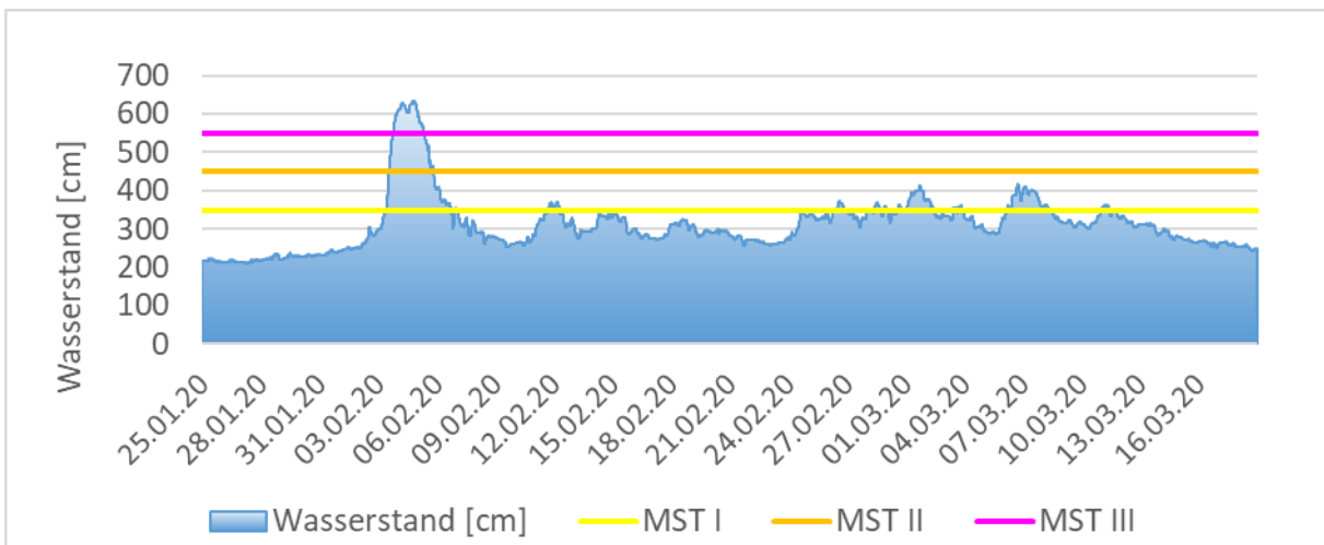
Abbildung 21: Wasserstand und Meldestufenüberschreitungen am Pegel Rockenau / Neckar 25. Januar bis 18. März 2020. Meldestufe 1 = 350 cm (gelbe Linie), Meldestufe 2 = 450 cm (orangefarbene Linie), Meldestufe 3 = 550 cm (pinke Linie)
