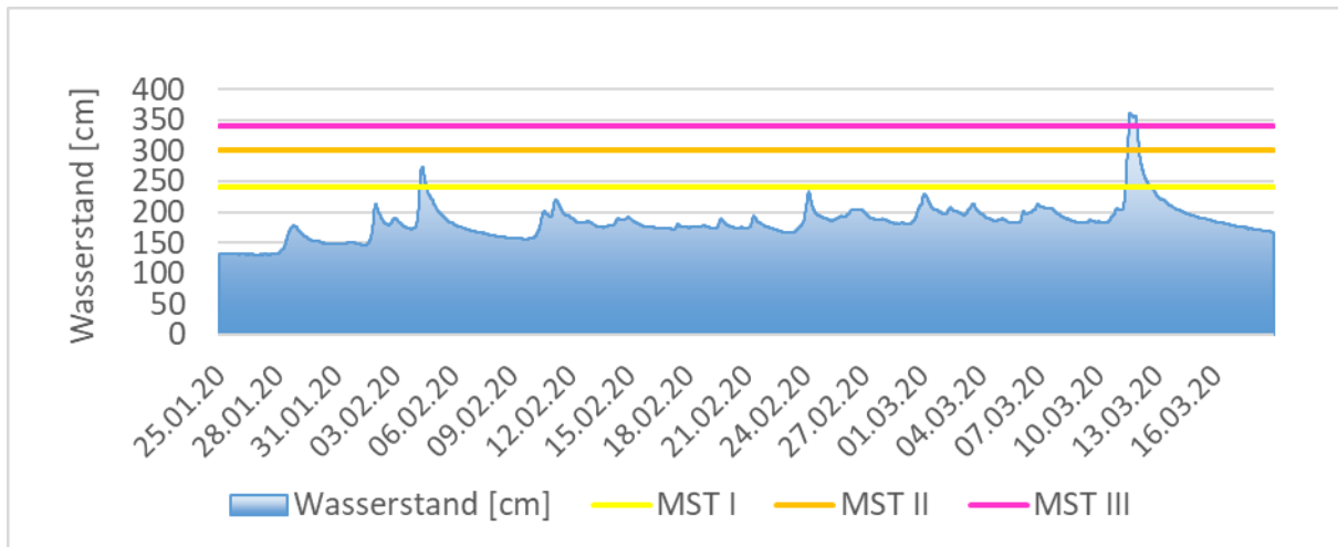
Abbildung 15: Wasserstand und Meldestufenüberschreitungen am Pegel Philippsthal / Ulster 25. Januar bis 18. März 2020. Meldestufe 1 = 240 cm (gelbe Linie), Meldestufe 2 = 300 cm (orangefarbene Linie), Meldestufe 3 = 340 cm (pinke Linie)
