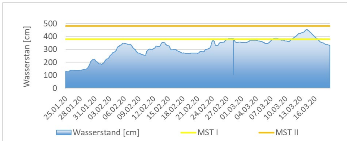
Abbildung 17: Wasserstand und Meldestufenüberschreitungen am Pegel Bad Karlshafen / Weser 25. Januar bis 18. März 2020. Meldestufe 1 = 380cm (gelbe Linie), Meldestufe 2 = 480 cm (orangefarbene Linie), Meldestufe 3 = 500 cm (nicht in Grafik zu sehen)
