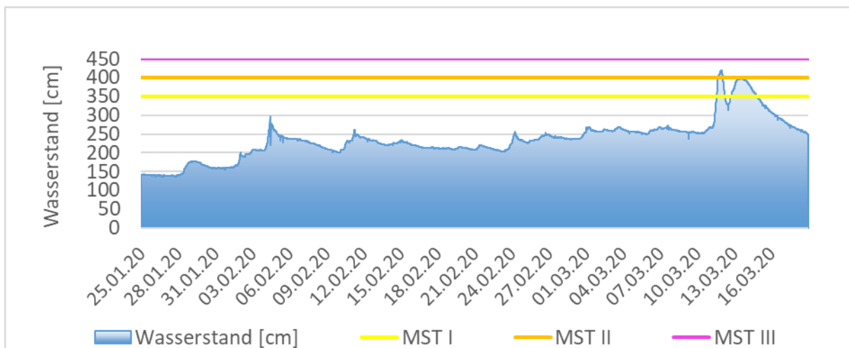
Abbildung 16: Wasserstand und Meldestufenüberschreitungen am Pegel Heimboldshausen / Werra 25. Januar bis 18. März 2020. Meldestufe 1 = 350 cm (gelbe Linie), Meldestufe 2 = 400 cm (orangefarbene Linie), Meldestufe 3 = 450 cm (pinke Linie)
