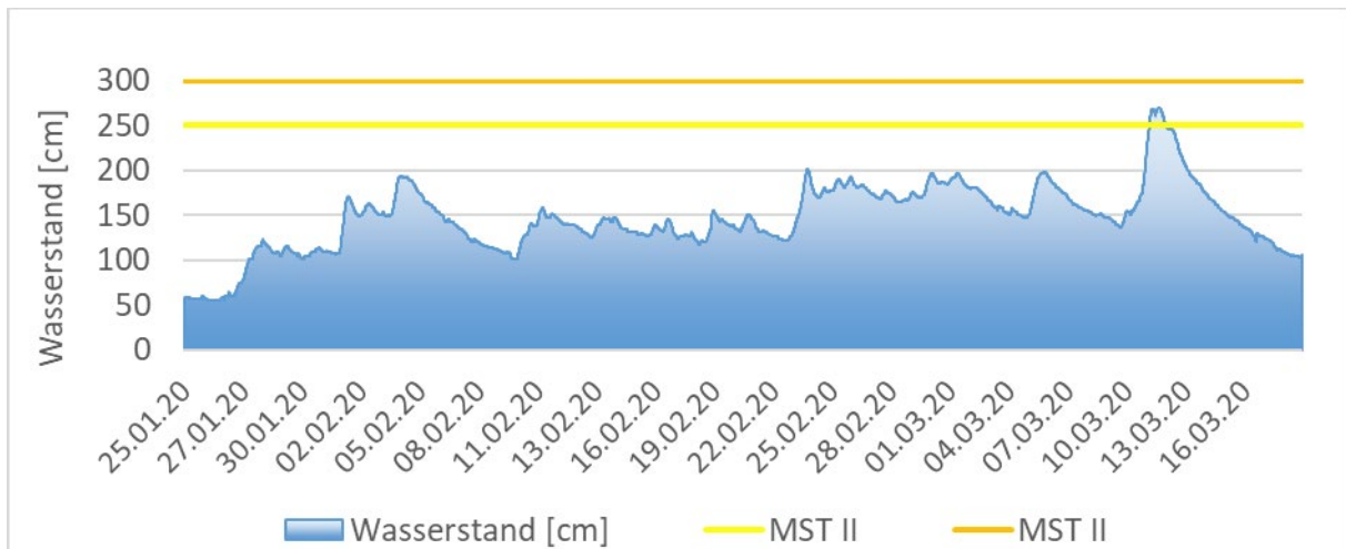
Abbildung 9: Wasserstand und Meldestufenüberschreitungen am Pegel Aßlar/ Dill 25. Januar bis 18. März 2020. Meldestufe 1 = 250 cm (gelbe Linie), Meldestufe 2 = 300 cm (orangefarbene Linie), Meldestufe 3 = 350 cm (nicht in Grafik zu sehen)
