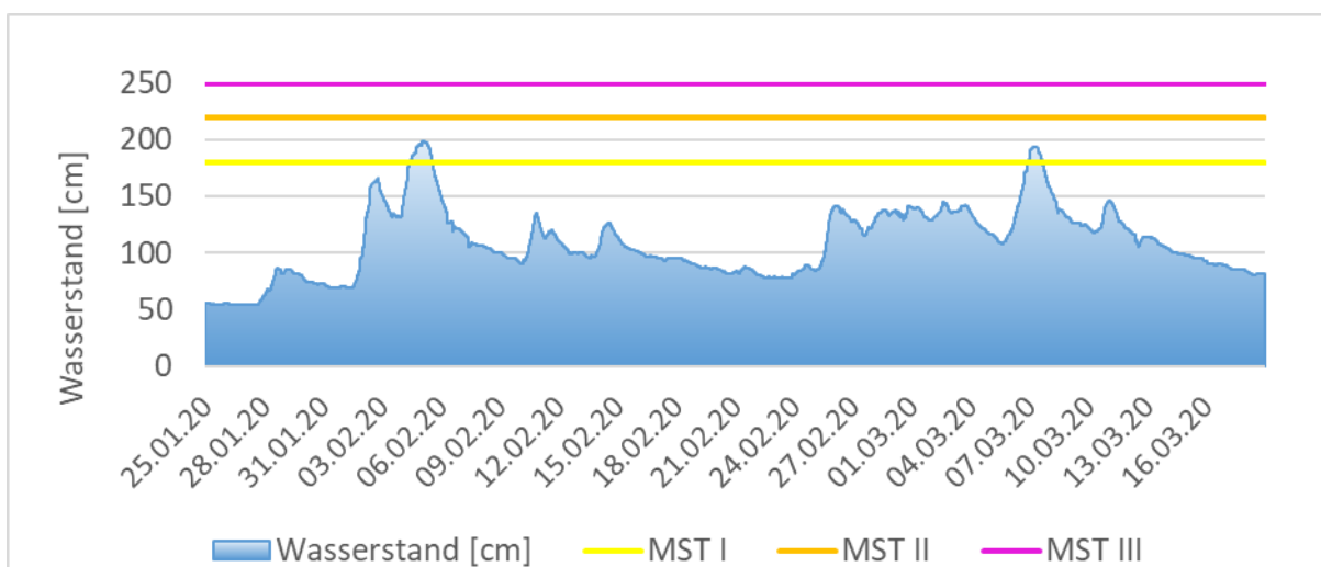
Abbildung 19: Wasserstand und Meldestufenüberschreitungen am Pegel Harreshausen / Gersprenz 25. Januar bis 18. März 2020. Meldestufe 1 = 180 cm (gelbe Linie), Meldestufe 2 = 220 cm (orangefarbene Linie), Meldestufe 3 = 250 cm (pinke Linie)
