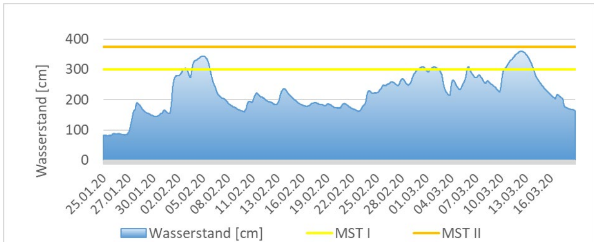
Abbildung 20: Wasserstand und Meldestufenüberschreitungen am Pegel Gelnhausen / Kinzig 25. Januar bis 18. März 2020. Meldestufe 1 = 300cm (gelbe Linie), Meldestufe 2 = 375 cm (orangefarbene Linie), Meldestufe 3 = 460 cm (nicht in Grafik zu sehen)
