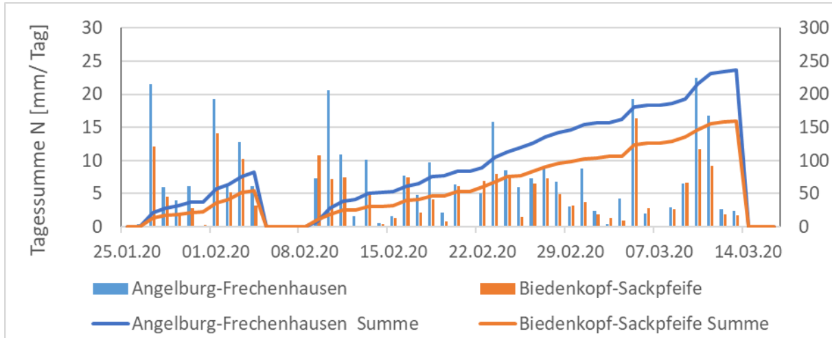
Abbildung 4: Tagesniederschlagssummen im Rothaargebirge
