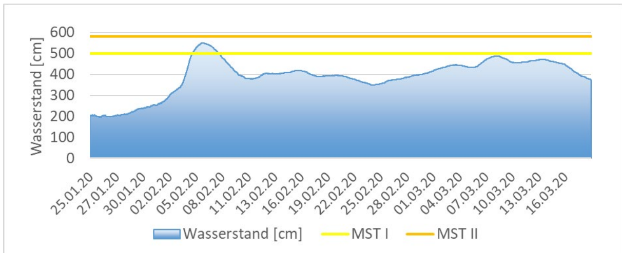
Abbildung 24: Wasserstand und Meldestufenüberschreitungen am Pegel Mainz / Rhein 25. Januar bis 18. März 2020. Meldestufe 1 = 500cm (gelbe Linie), Meldestufe 2 = 580 cm (orangefarbene Linie), Meldestufe 3 = 650 cm (nicht in Grafik zu sehen)
