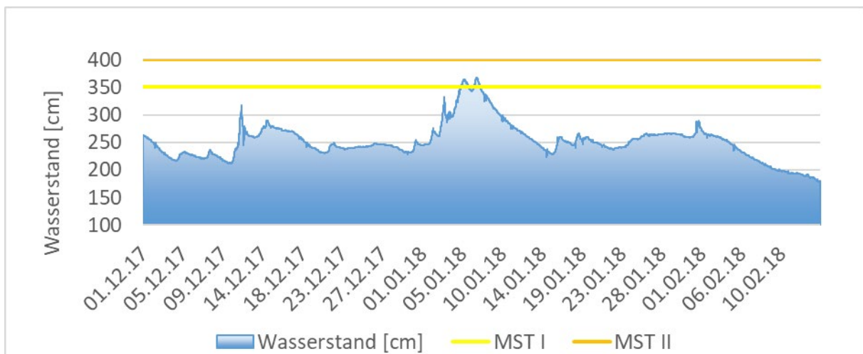
Abbildung 37: Wasserstand am Pegel Heimbaldshausen / Werra. Meldestufe 1 = 350 cm (gelbe Linie), Meldestufe 2 = 400 cm (orangefarbene Linie), Meldestufe 3 = 450 cm (nicht in Grafik zu sehen)
