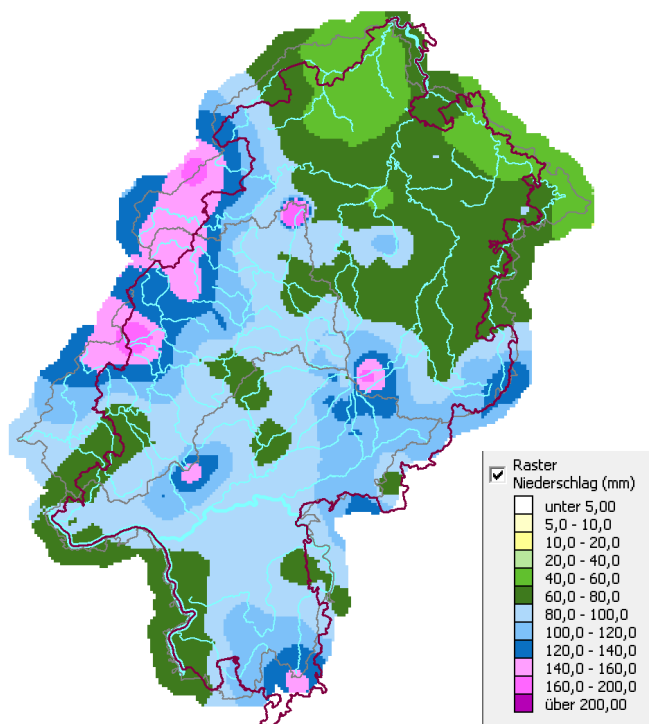
Abbildung 2: Niederschlagssummen 1. bis 31. Dezember 2017 (LARSIM)
