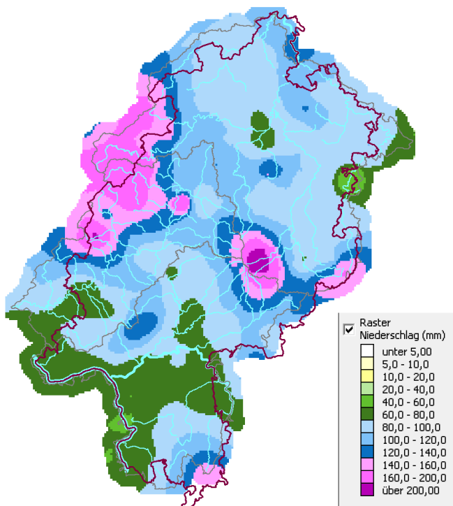
Abbildung 3: Niederschlagssumme 1. bis 31. Januar 2018 (LARSIM)
