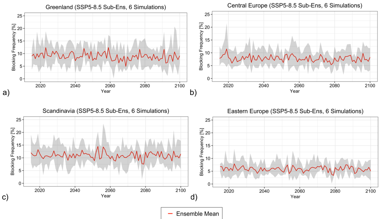
Abbildung 11: Zeitliche Entwicklung der blocking -Frequenz in verschiedenen Regionen im europäisch-atlantischen Raum im gewählten CMIP6-Sub-Ensemble des SSP5-8.5-Szenarios. Die rote Linie kennzeichnet das Ensemble-Mittel, der graue Bereich die Bandbreite des Ensembles.
