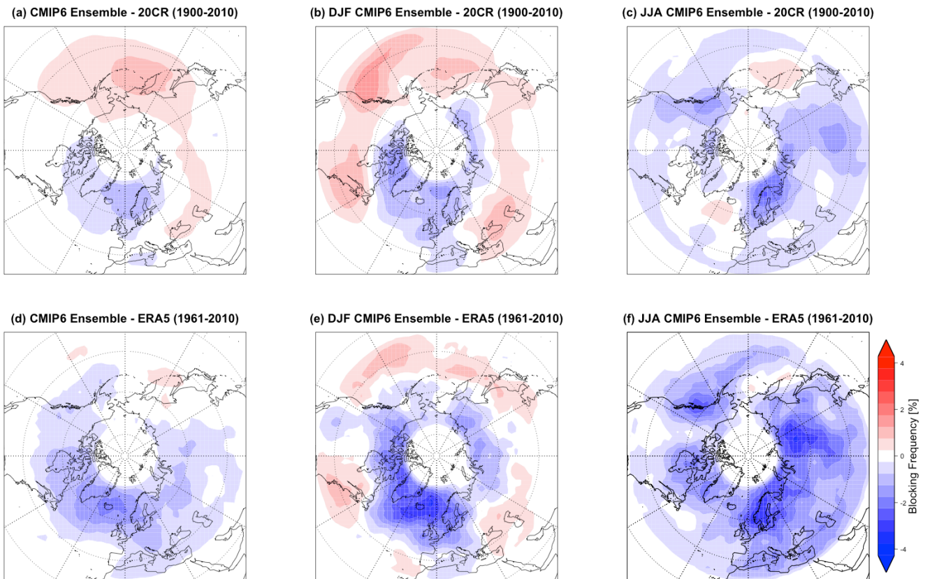
Abbildung 5: Abweichung der blocking -Frequenz im CMIP6-Ensemble-Mittel von der 20CR-Reanalyse im Zeitraum 1900-2010 (a-c) und von der ERA5-Reanalyse im Zeitraum 1961-2010 (d-f), bezogen auf das ganze Jahr (a,d), Winter (b,e) und Sommer (c,f).
