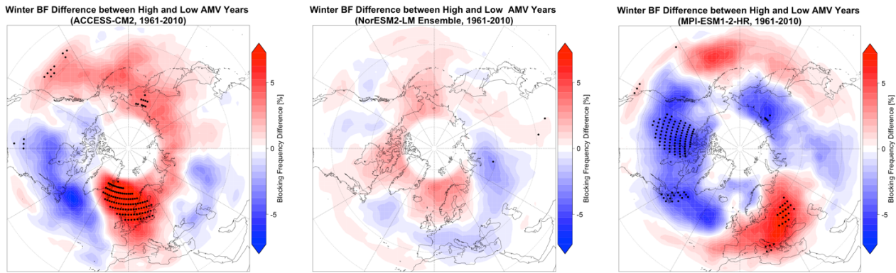
Abbildung 16: Differenz der Winter- blocking -Frequenz zwischen Jahren mit positiver und negativer AMV (1961-2010) in ausgewählten CMIP6-Simulationen. Punkte kennzeichnen Signifikanz auf dem 5%-Niveau.
