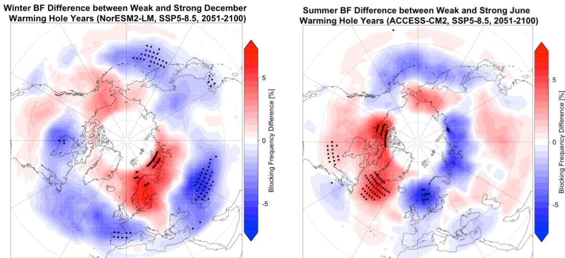
Abbildung 25: Differenz der Winter- blocking -Frequenz zwischen Jahren mit schwach und stark ausgeprägtem Erwärmungsloch im Dezember (2051-2100) in NorESM2-LM (links) und Differenz der Sommer- blocking -Frequenz zwischen Jahren mit schwach und stark ausgeprägtem Erwärmungsloch im Juni in ACCESS-CM2 (rechts), jeweils im SSP5-8.5-Szenario. Punkte kennzeichnen Signifikanz auf dem 5%-Niveau.
