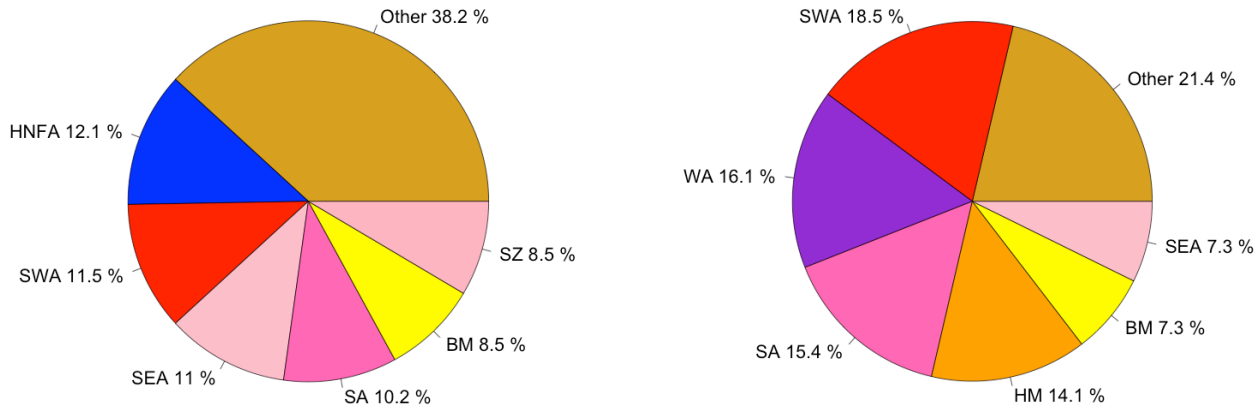
Abbildung 52: Häufigkeit der Wetterlagen nach Hess & Brezowsky an Tagen mit Hitzewelle im Sommerhalbjahr (April-September, 1961-2010) in der Mitte Deutschlands in ERA5-Reanalyse (links) und NorESM2-LM (rechts). Wetterlagen mit einer Häufigkeit unter 5% werden zur besseren Übersichtlichkeit unter „Other“ zusammengefasst.
