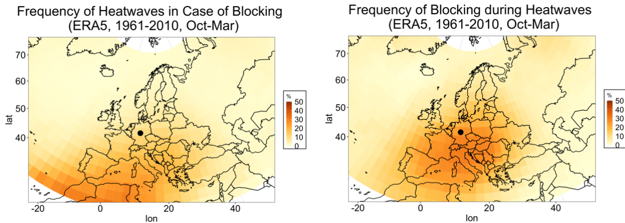
Abbildung 55: Häufigkeit von Hitzewellen während blocking (links) und von blocking während Hitzewellen (rechts) am markierten Punkt im Winterhalbjahr (Oktober-März, 1961-2010) in ERA5.
