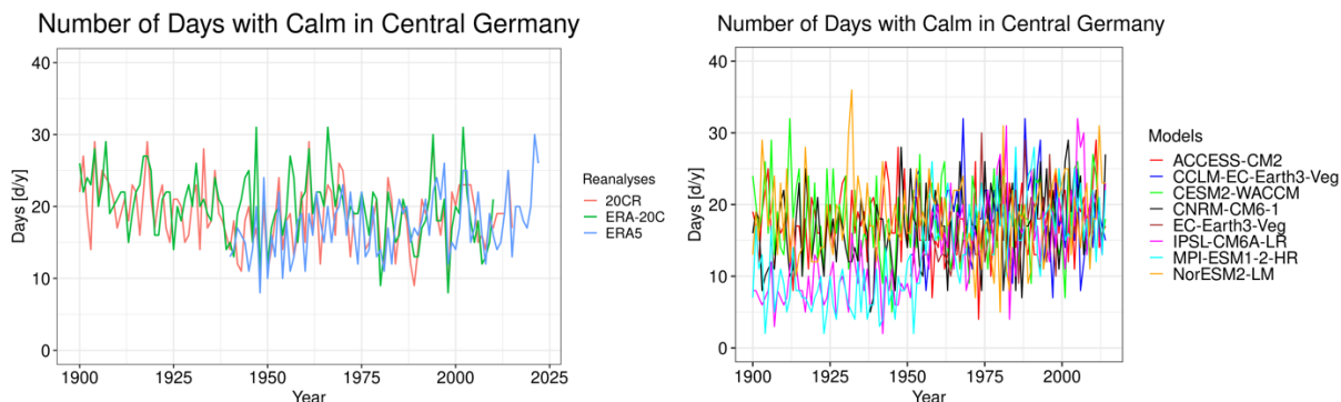
Abbildung 50: Anzahl der Flaute-Tage pro Jahr in Reanalysen (links) und CMIP6-Simulationen (rechts) in der Mitte Deutschlands (51°N, 10°O). Aufgrund unterschiedlicher Gitter der Modelle können die genauen Koordinaten des gewählten Punktes leicht abweichen.
