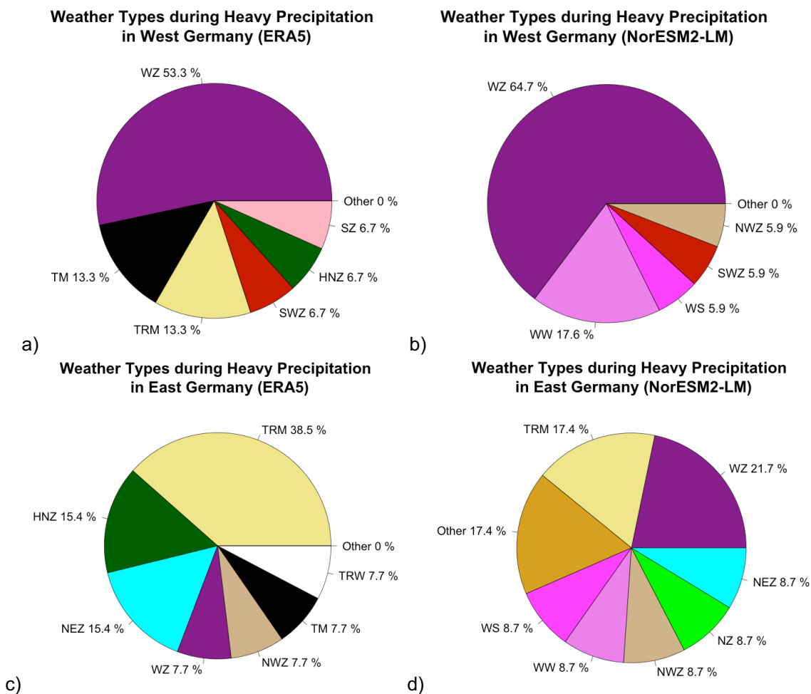
Abbildung 56: Wie Abbildung 52, aber für Tage mit Starkregen in West- und Ostdeutschland (1961-2010) in ERA5-Reanalyse (a,c) und NorESM (b,d).
