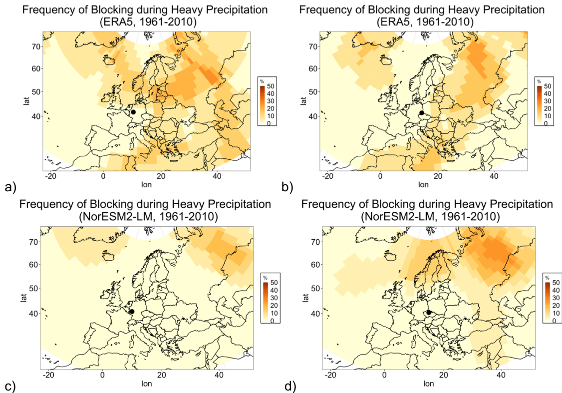
Abbildung 57: Häufigkeit von blocking während Starkregen in Westdeutschland (links) und Ostdeutschland (rechts) (1961-2010) in ERA5 (oben) bzw. NorESM (unten).
