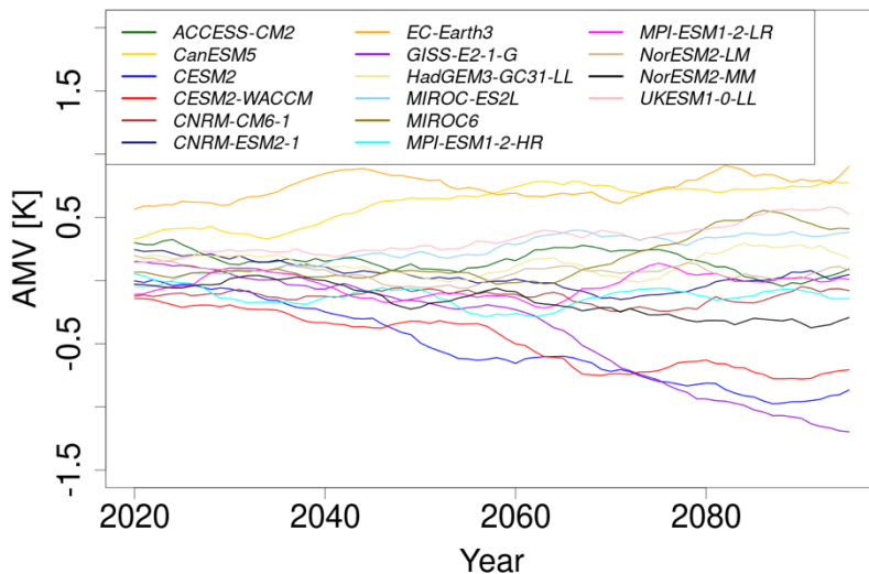
Abbildung 17: AMV in SSP5-8.5-Szenario. Zur besseren Übersichtlichkeit wird nur das 11-jährige gleitende Mittel gezeigt.
