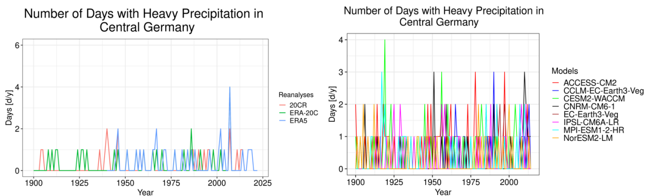
Abbildung 46: Anzahl der Starkregen-Tage pro Jahr in Reanalysen (links) und CMIP6-Simulationen (rechts) in der Mitte Deutschlands (51°N, 10°O). Aufgrund unterschiedlicher Gitter der Modelle können die genauen Koordinaten des gewählten Punktes leicht abweichen.
