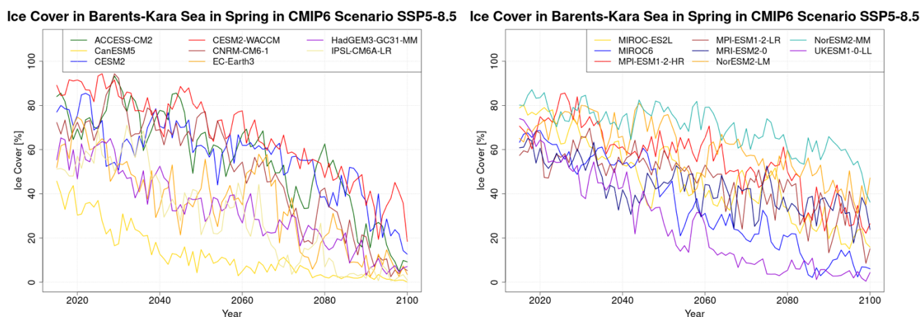
Abbildung 38: Wie Abbildung 36, aber in CMIP6-Simulationen einer SSP5-8.5-Zukunft.
