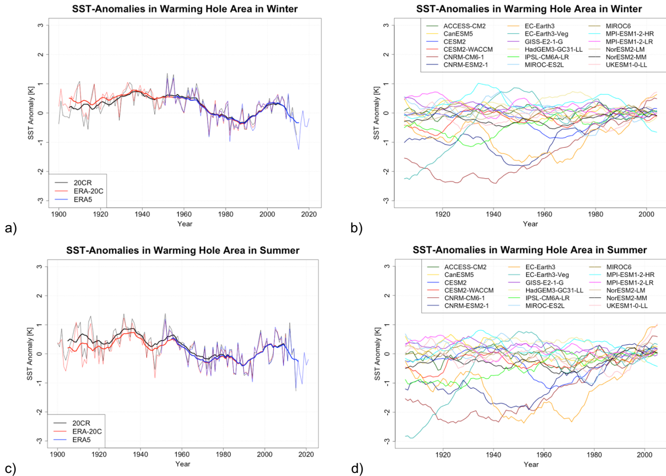
Abbildung 20: Differenz zwischen Abweichung der SST im Erwärmungsloch ( 45^{\circ} - 60^{\circ} N, 50^{\circ} - 15^{\circ} W) vom Mittel des Zeitraums 1981-2010 und Abweichung der globalen SST vom Mittel des Zeitraums 1981-2010 in den Monaten Dezember bis Februar (a,b) und Juni bis August (c,d) in Reanalysen (a,c) und CMIP6-Simulationen (b,d). Zur besseren Übersichtlichkeit wird bei den Simulationen nur das 11-jährige gleitende Mittel gezeigt.
