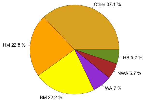
Abbildung 61: Wie Abbildung 52, aber für Tage mit Flaute (1961-2010) in der Mitte Deutschlands in ERA5-Reanalyse (links) und NorESM (rechts).
