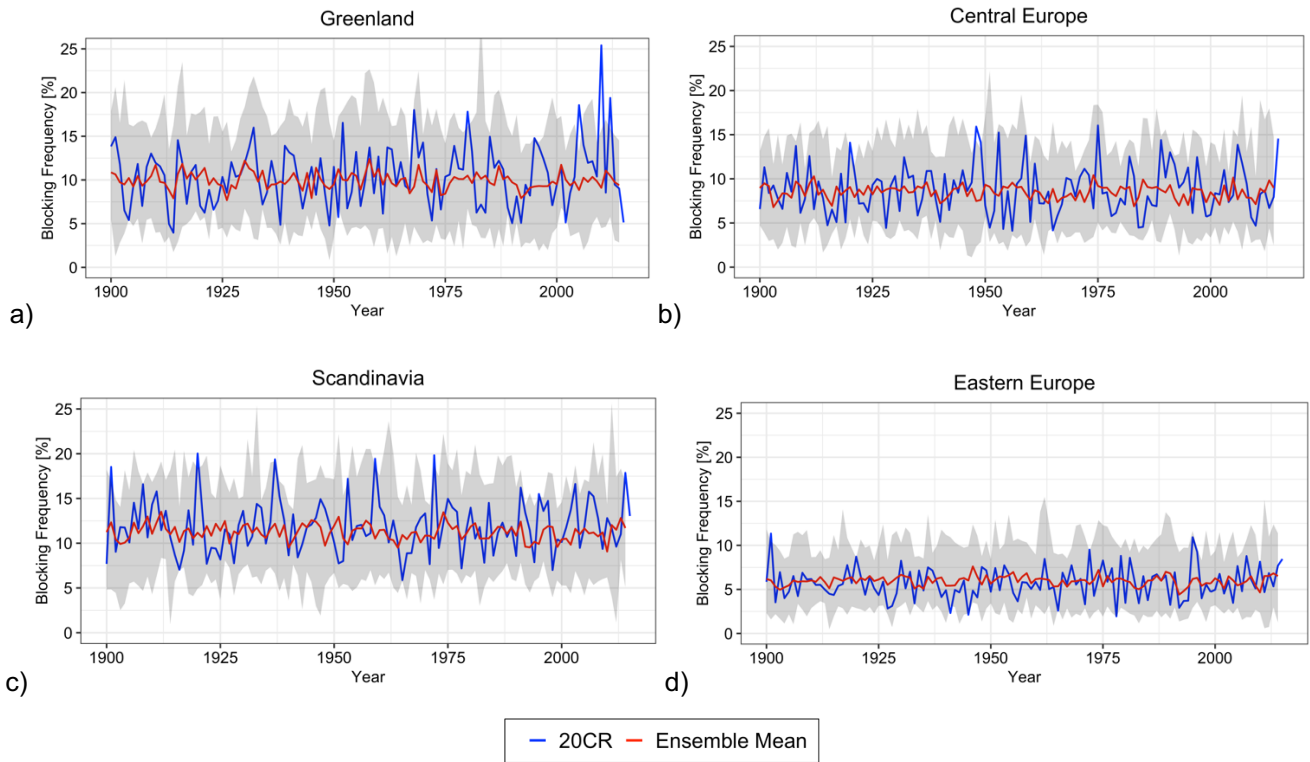
Abbildung 6: Zeitliche Entwicklung der blocking -Frequenz in verschiedenen Regionen im europäisch-atlantischen Raum. Die rote Linie kennzeichnet das CMIP6-Ensemble-Mittel, die blaue die 20CR-Reanalyse, der graue Bereich die Bandbreite des Ensembles.
