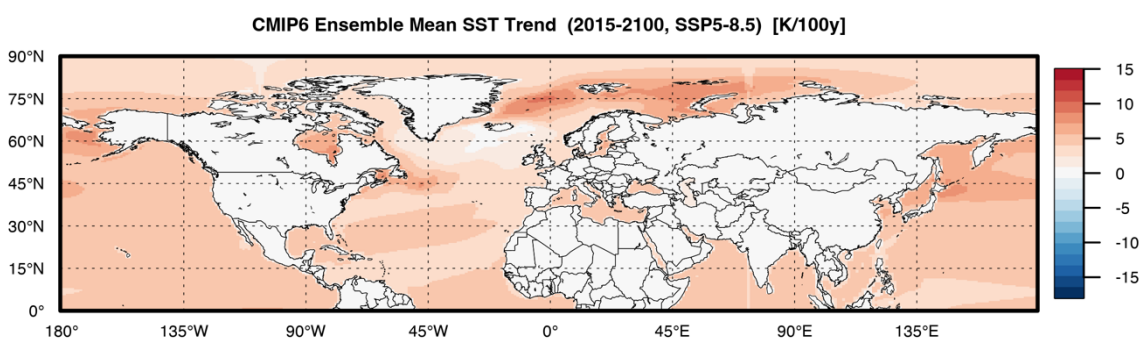
Abbildung 23: SST-Trend in Nordhemisphäre (2015-2100), hochgerechnet auf 100 Jahre in SSP5-8.5-Szenario im Ensemblemittel.
