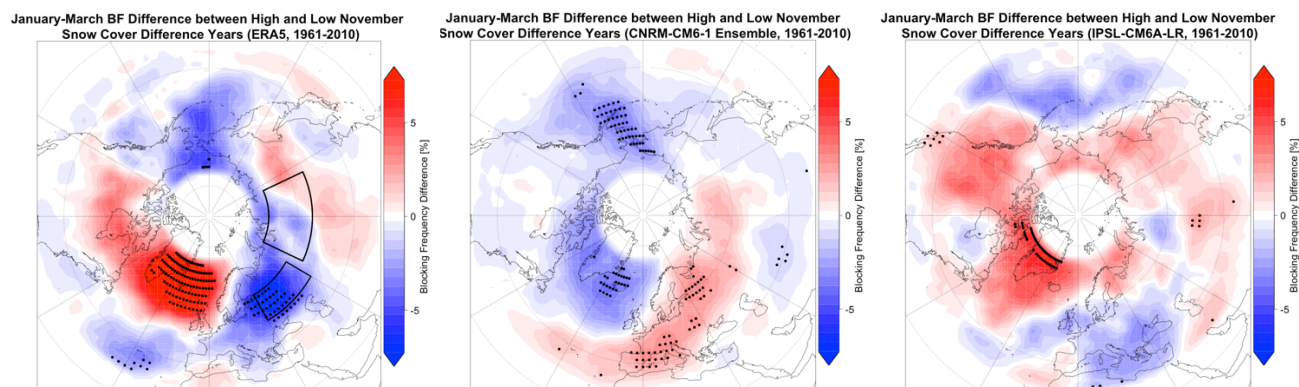
Abbildung 33: Differenz der blocking -Frequenz der Monate Januar bis März zwischen Jahren mit großen und kleinen Unterschieden der Schneebedeckung westlich ( 50^{\circ} - 60^{\circ} N, 30^{\circ} - 60^{\circ} O) und östlich ( 55^{\circ} - 70^{\circ} N, 65^{\circ} - 115^{\circ} O) des im November in ERA5 (links), CNRM-CM6-1 (Mitte) sowie IPSL-CM6A-LR (rechts). Punkte kennzeichnen Signifikanz auf dem 5%-Niveau. Die beiden Boxen in der linken Abbildung kennzeichnen die Regionen, zwischen denen die Differenz der Schneebedeckung berechnet wird.
