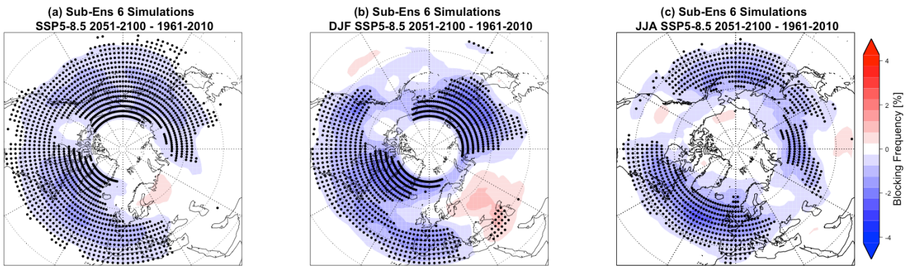
Abbildung 10: Änderung der blocking -Frequenz im Mittel des gewählten CMIP6-Sub-Ensembles zwischen den Zeiträumen 2051-2100 und 1961-2010 im SSP5-8.5-Szenario im ganzen Jahr (a), Winter (b) und Sommer (c). Punkte kennzeichnen Signifikanz auf dem 5%-Niveau.
