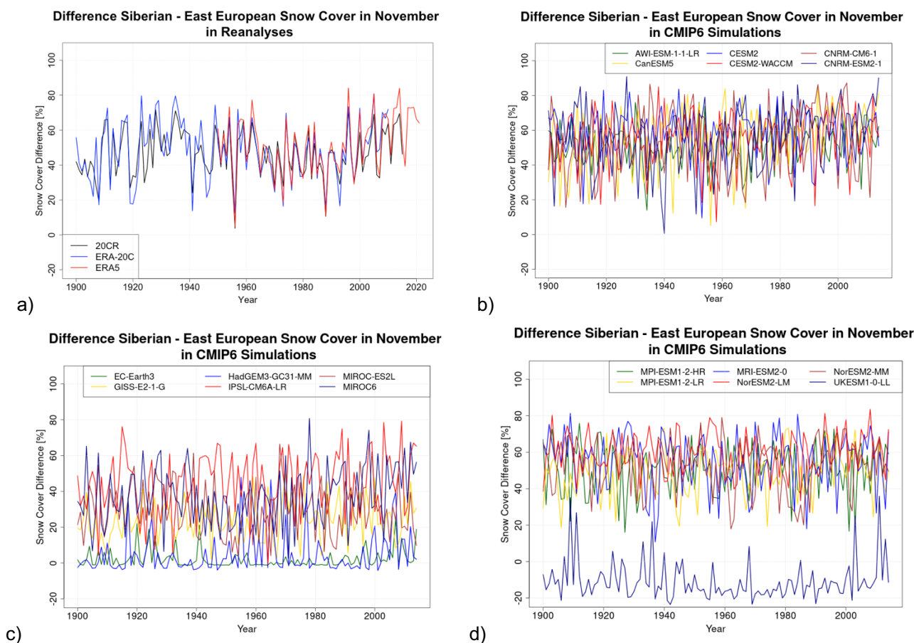
Abbildung 32: Differenz in der mittleren Schneebedeckung westlich (50°-60°N, 30°-60°O) und östlich (55°-70°N, 65°-115°O) des Urals in Reanalysen (a) und CMIP6-Simulationen (b-d) im November. Zur besseren Übersichtlichkeit werden die Zeitserien der CMIP6-Simulationen in 3 Graphen gezeigt.
