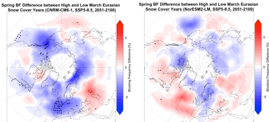
Abbildung 31: Differenz der Frühlings- blocking -Frequenz zwischen Jahren mit hoher und niedriger Schneebedeckung in Eurasien im März (2051-2100) in CNRM-CM6-1 (links) und NorESM2-LM im SSP5-8.5-Szenario. Punkte kennzeichnen Signifikanz auf dem 5%-Niveau.
