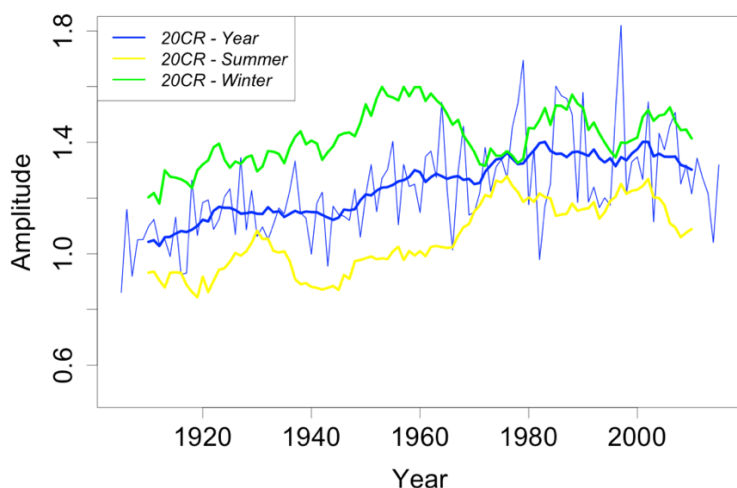
Abbildung 26: Amplitude der Madden-Julian-Oszillation (nach Oliver und Thompson, 2012) in 20CR. Die dickeren Linien kennzeichnen das gleitende 11-jährige Mittel.
