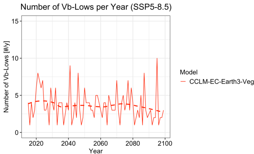
Abbildung 49: Anzahl Vb-Tiefdruckgebiete pro Jahr in CCLM-EC-Earth3-Veg im SSP5-8.5-Szenario.
