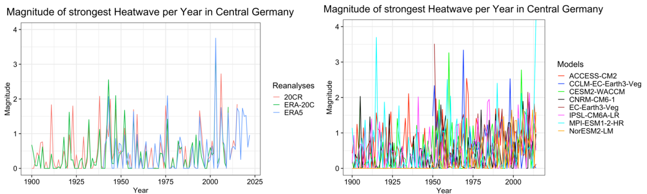
Abbildung 42: Wie Abbildung 41, aber für die Magnitude der stärksten Hitzewelle eines Jahres.
