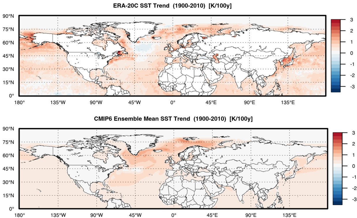
Abbildung 19: SST-Trend in Nordhemisphäre (1900-2010), hochgerechnet auf 100 Jahre in ERA-20C-Reanalyse (oben) und CMIP6-Ensemblemittel (unten).
