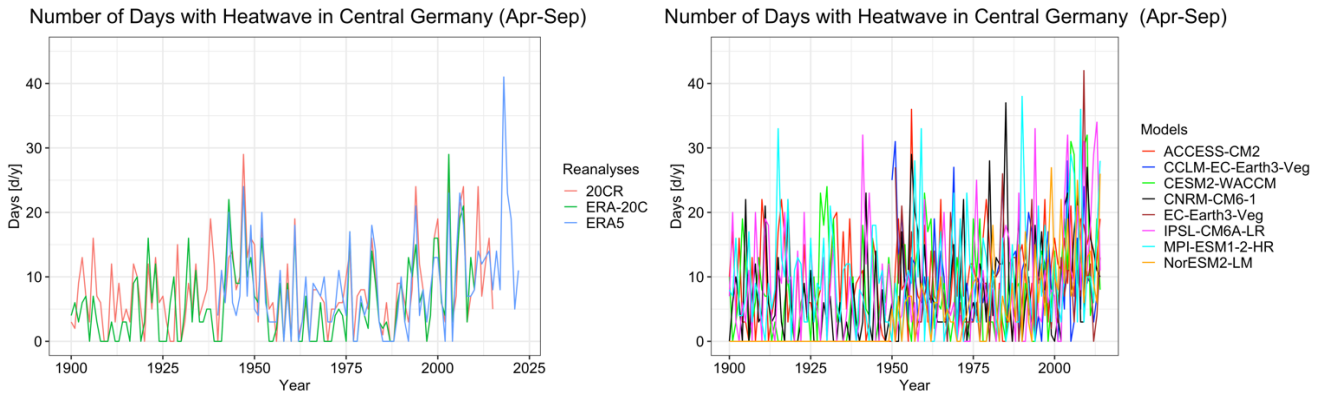
Abbildung 41: Anzahl der Tage mit Hitzewellen im Sommerhalbjahr (April bis September) in Reanalysen (links) und CMIP6-Simulationen (rechts) in der Mitte Deutschlands (51°N, 10°O). Aufgrund unterschiedlicher Rechengitter der Modelle können die Koordinaten des gewählten Punktes leicht abweichen.
