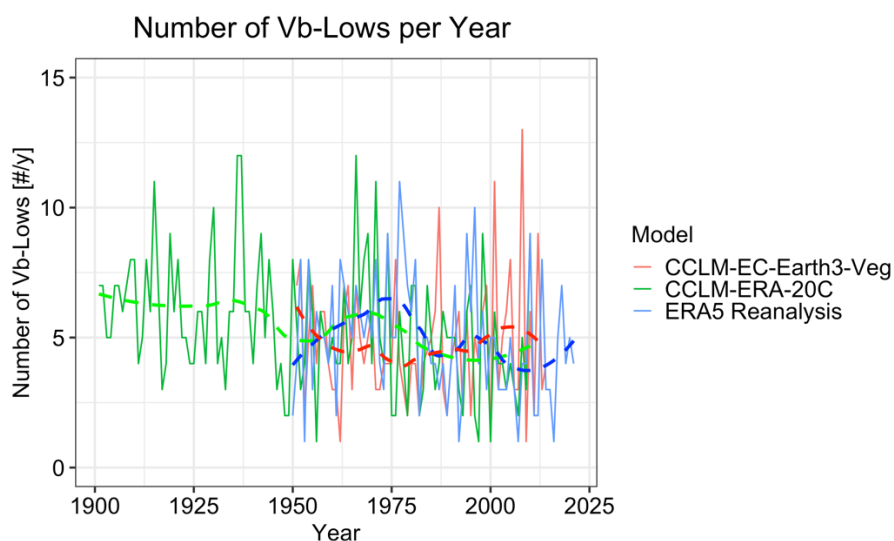
Abbildung 48: Anzahl Vb-Tiefdruckgebiete pro Jahr in ERA5, CCLM-ERA-20C und CCLM-EC-Earth3-Veg.
