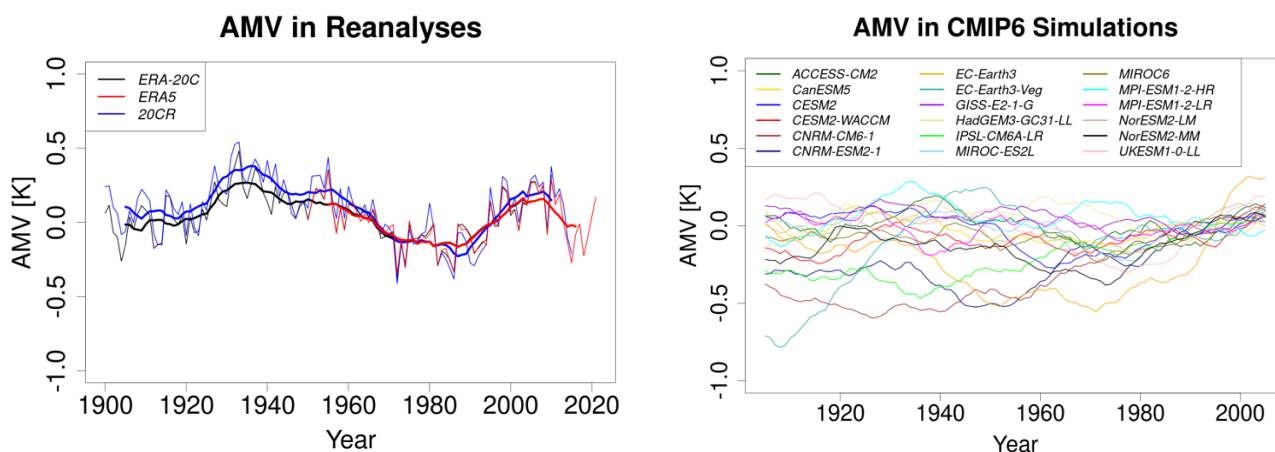
Abbildung 14: AMV in Reanalysen (links) und CMIP6-Simulationen (rechts). Zur besseren Übersichtlichkeit wird bei den CMIP6-Simulationen nur das 11-jährige gleitende Mittel gezeigt.
