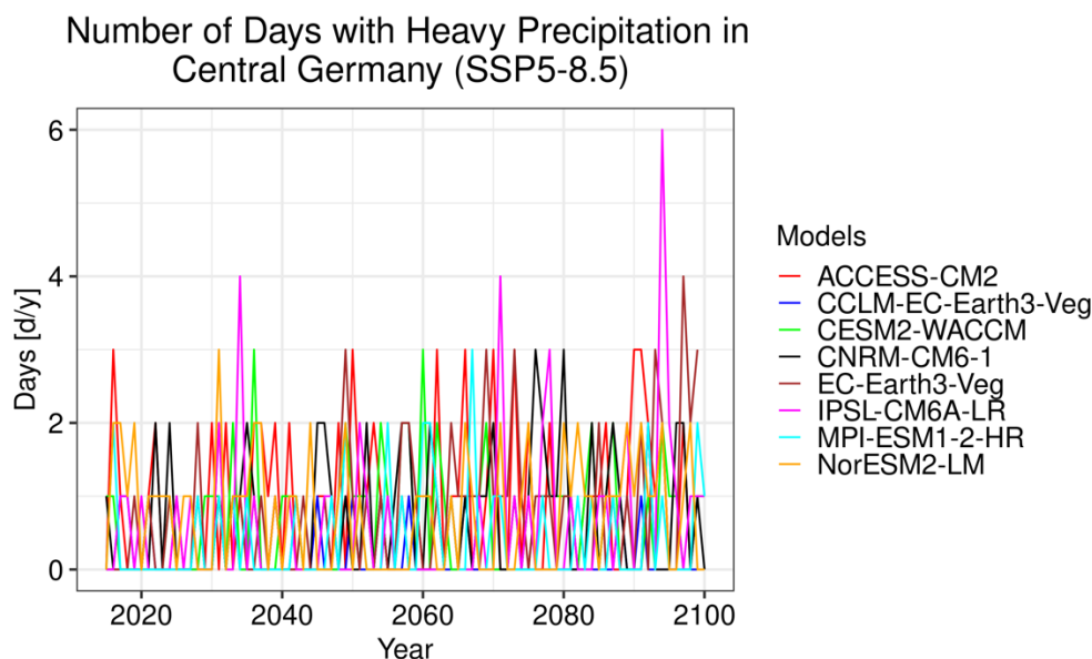
Abbildung 47: Wie Abbildung 46, aber im CMIP6-Szenario SSP5-8.5.
