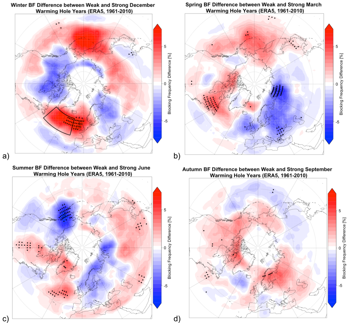
Abbildung 21: Differenz der saisonalen blocking -Frequenz zwischen Jahren mit schwach und stark ausgeprägtem Erwärmungsloch im ersten Monat einer Jahreszeit (1961-2010) in ERA5-Reanalyse. Punkte kennzeichnen Signifikanz auf dem 5%-Niveau. (a) Dezember-Winter, (b) März-Frühling, (c) Juni-Sommer, (d) September-Herbst. Die Box in (a) kennzeichnet die Region, in der die SST-Anomalien betrachtet werden.
