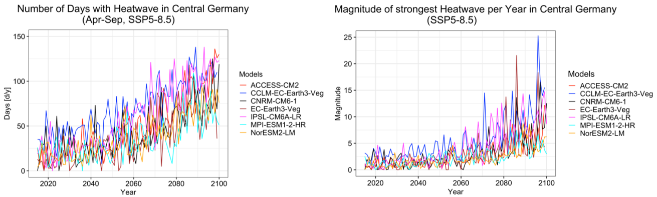
Abbildung 43: Wie Abbildung 41, aber für Anzahl der Tage mit Hitzewellen im Sommerhalbjahr (April bis September, links) und Magnitude der stärksten Hitzewelle eines Jahres (rechts) im CMIP6-Szenario SSP5-8.5.
