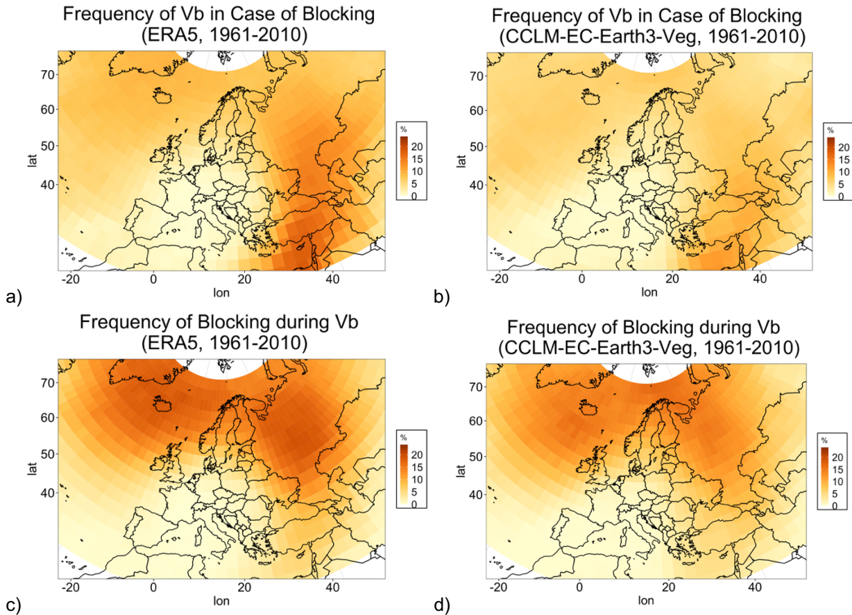
Abbildung 58: Häufigkeit von Vb-Tiefs im Fall von blocking (1961-2010) in ERA5 (a) und CCLM-EC-Earth3-Veg (b). Häufigkeit von blocking während Vb in ERA5 (c) und CCLM-EC-Earth3-Veg (d).
