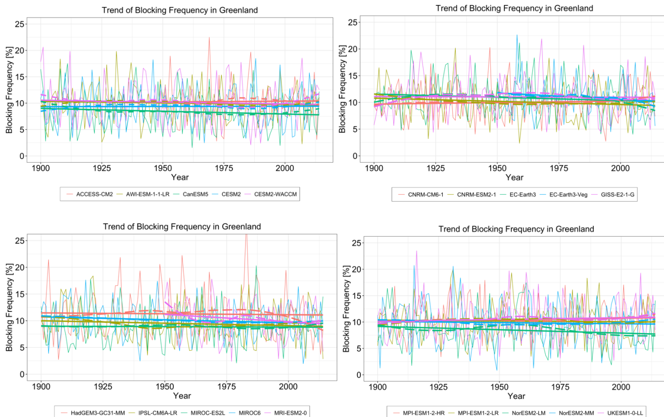
Abbildung 7: Zeitserien der jährlichen blocking -Frequenz in Grönland in CMIP6-Simulationen. Zur besseren Übersichtlichkeit sind die Ergebnisse auf vier Graphen aufgeteilt.
