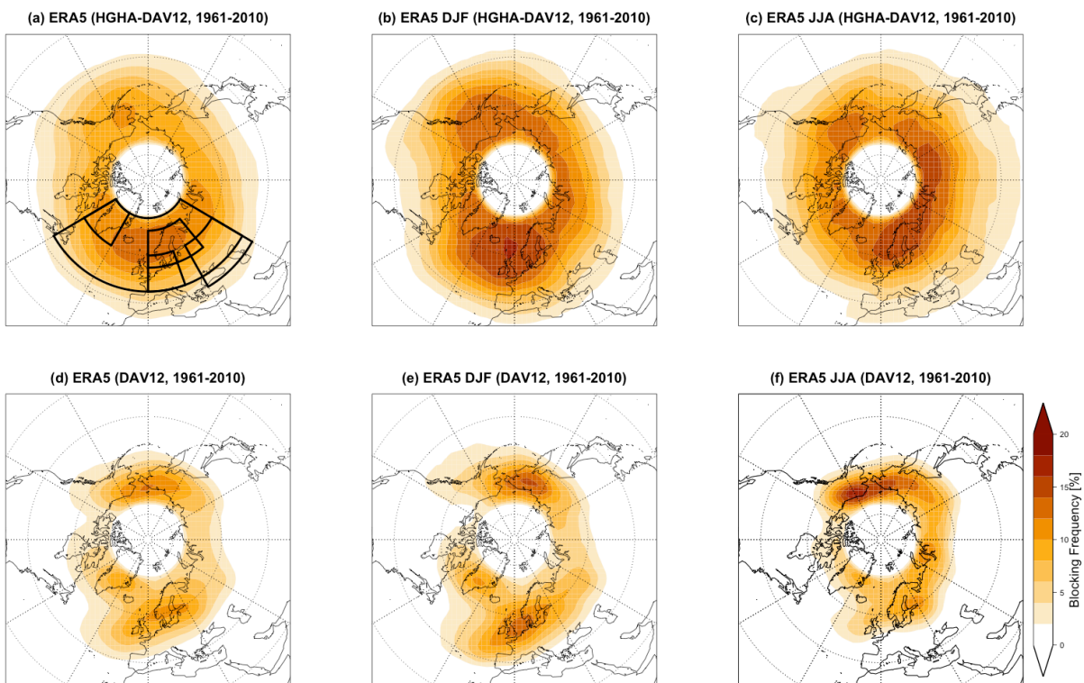
Abbildung 1: Mittlere blocking -Frequenz in ERA5 im Zeitraum 1961-2010 unter Verwendung des HGHA-DAV12 (a-c) und DAV12 (d-f). Die Mittelwerte zeigen jährliche (a,d) bzw. saisonale blocking -Frequenz für den Winter (b,e) sowie den Sommer (c,f). Die kleinen Boxen in (a) zeigen die Regionen, für die Zeitserien der blocking -Frequenz erstellt wurden, die große Box den Ausschnitt, für den Anzahl, Dauer und räumliche Ausdehnung der blocking -Ereignisse untersucht wurden.
