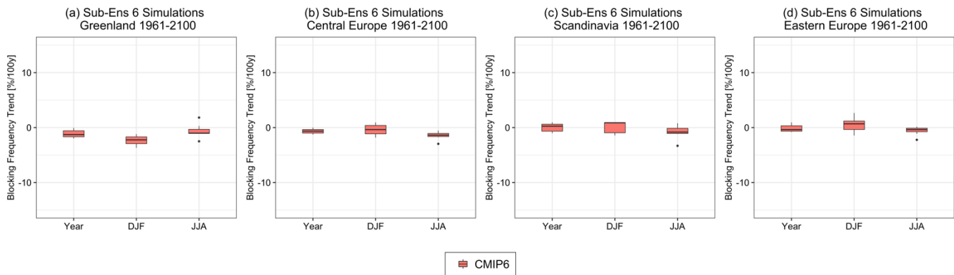
Abbildung 13: Boxplots der blocking -Trends (jährliche, winterliche und sommerliche Trends) in den Regionen in den Simulationen des CMIP6-Subensembles im Szenario SSP5-8.5. Die drei horizontalen Linien zeigen das erste und dritte Quartil, sowie den Median. Striche zeigen den Ensemble-Range, sind aber auf das 1,5-fache des Interquartilsabstands begrenzt. Trendwerte außerhalb dieses Bereichs sind durch Punkte gekennzeichnet.
