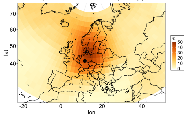
Abbildung 53: Häufigkeit von Hitzewellen im Fall von blocking und von blocking während Hitzewellen am markierten Punkt im Sommerhalbjahr (April-September, 1961-2010) in ERA5 (rechts).
