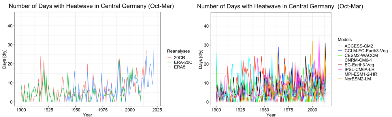
Abbildung 44: Wie Abbildung 41, aber für Anzahl der Tage mit Hitzewellen im Winterhalbjahr (Oktober bis März) in Reanalysen (links) und CMIP6-Simulationen (rechts).
