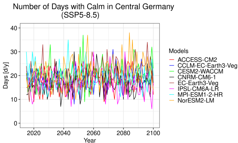
Abbildung 51: Wie Abbildung 50, aber im CMIP6-Szenario SSP5-8.5.
