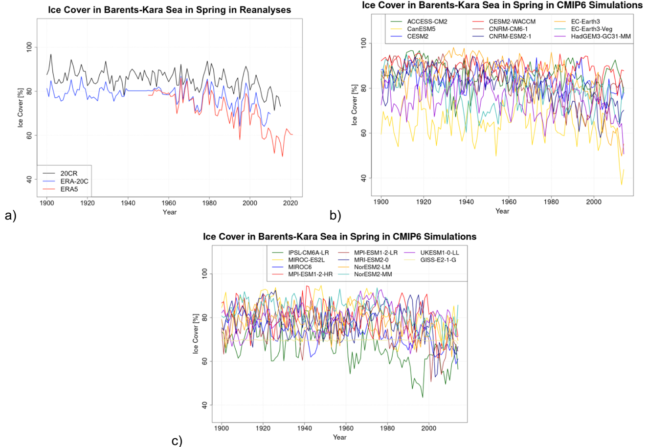
Abbildung 36: Eisbedeckung in der Barents-Karasee (68°-85°N, 25°-100°O) in den Monaten März bis Mai in Reanalysen (a) und CMIP6-Simulationen (b,c). Zur besseren Übersichtlichkeit werden die Zeitserien der CMIP6-Simulationen in 2 Graphen gezeigt.
