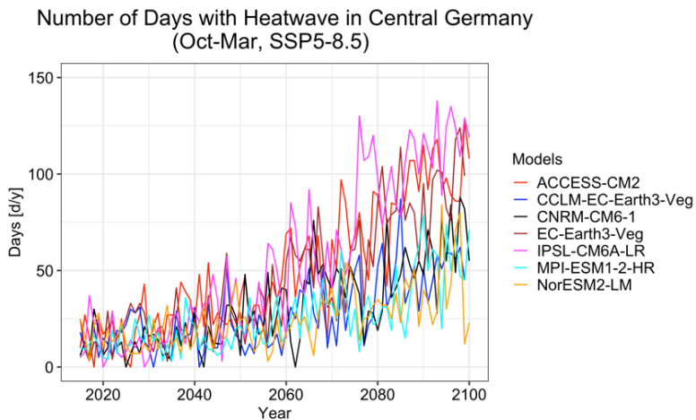
Abbildung 45: Wie Abbildung 41, aber für Anzahl der Tage mit Hitzewellen im Winterhalbjahr (Oktober bis März) im CMIP6-Szenario SSP5-8.5.
