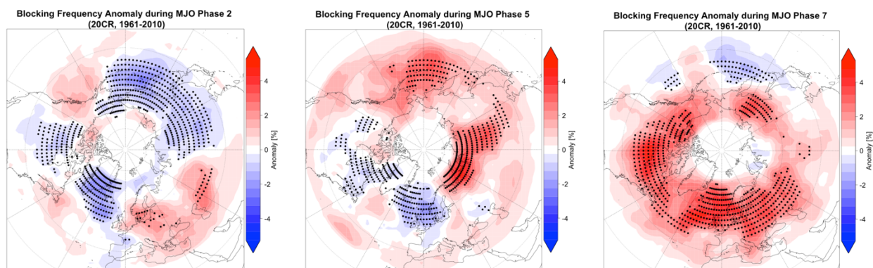
Abbildung 27: Abweichungen der blocking -Frequenz vom langjährigen Mittel (1961-2010) in 20CR-Reanalyse während MJO-Phasen 2 (links), 5 (Mitte) und 7 (rechts). Punkte kennzeichnen Signifikanz auf dem 5%-Niveau.
