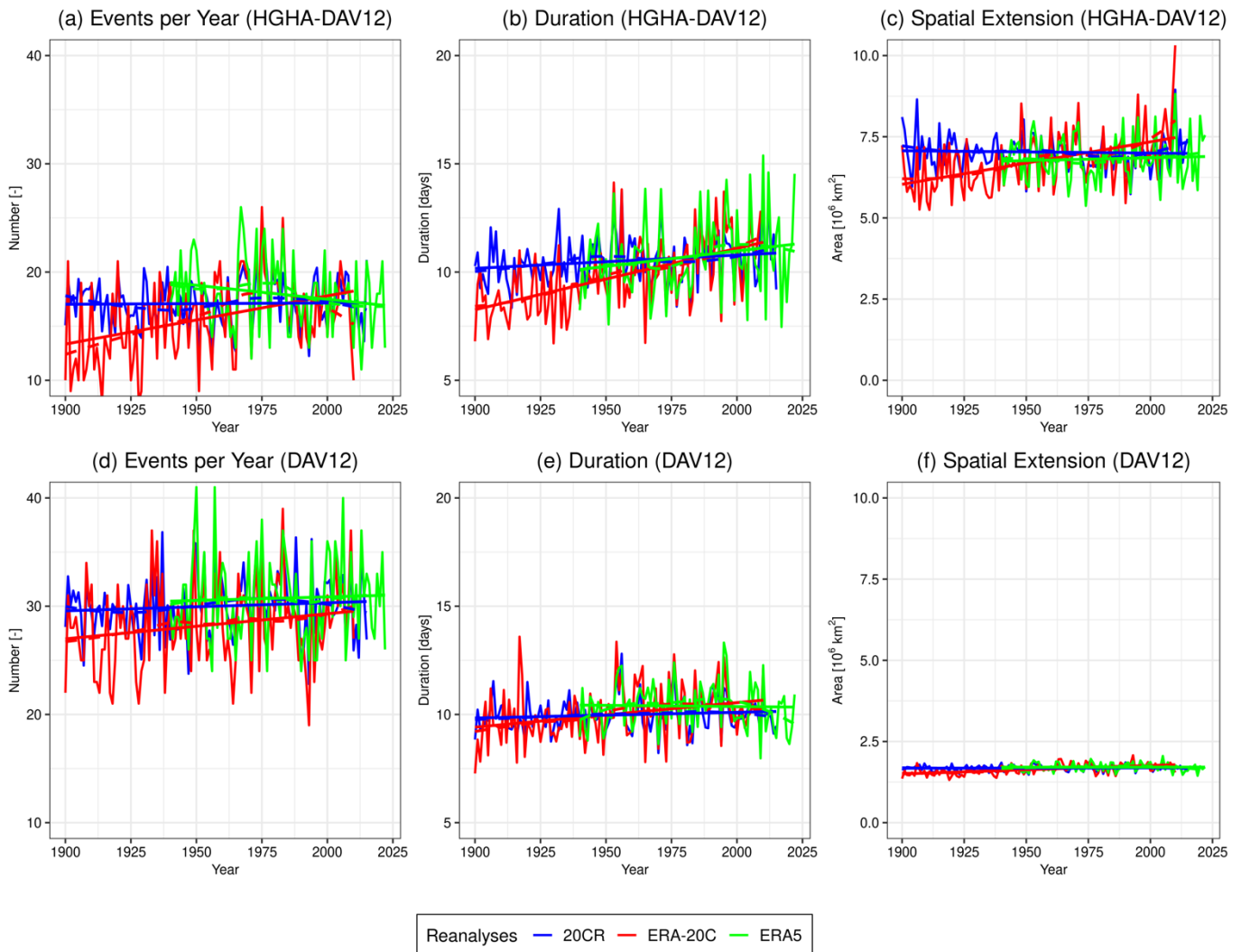
Abbildung 4: Zeitliche Entwicklung der Anzahl pro Jahr (a,d), der mittleren Dauer (b,e) und der mittleren räumlichen Ausdehnung (c,f) der blocking -Ereignisse mit HGHA-DAV12 (a-c) und DAV12 (d-f). Es wurden alle blocks in der Region zwischen 45° und 75°N sowie 60°W und 60°O berücksichtigt.
