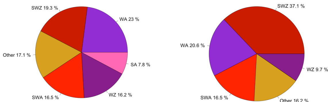
Abbildung 54: Wie Abbildung 52, aber für Tage mit Hitzewelle im Winterhalbjahr (Oktober-März, 1961-2010).
