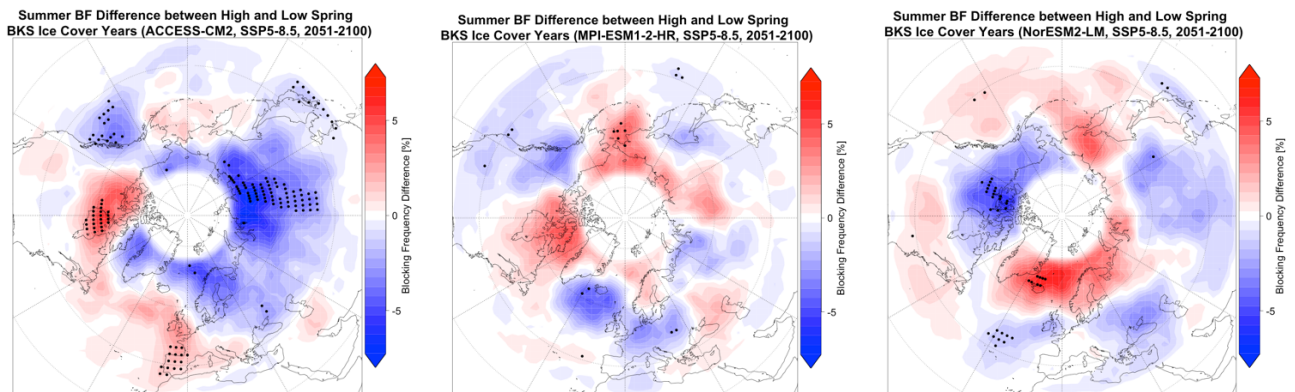
Abbildung 39: Wie Abbildung 37, aber in Simulationen mit ACCESS-CM2 (links), MPI-ESM1-2-HR (Mitte) und NorESM2-LM (rechts) einer SSP5-8.5-Zukunft.
