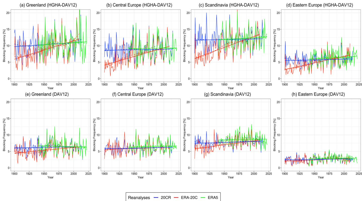
Abbildung 2: Zeitliche Entwicklung der jährlichen blocking -Frequenz in verschiedenen Regionen (s. Abbildung 1a, (a,e) Grönland, (b,f) Mitteleuropa, (c,g) Skandinavien, (d,h) Osteuropa) in Abhängigkeit vom blocking -Index (a-d) HGHA-DAV12, (e-h) DAV12). Dicke Linien zeigen lineare, gestrichelte Linien gleitende Trends.
