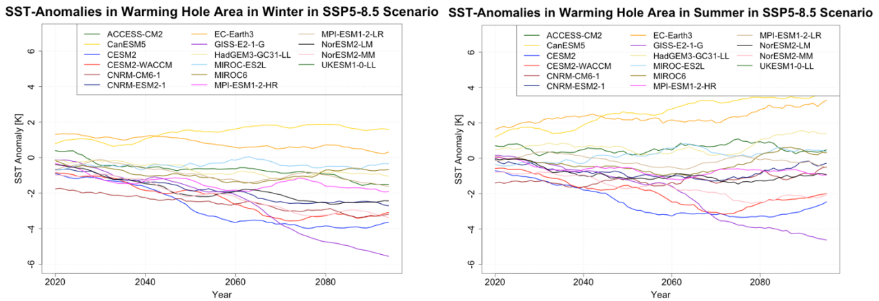
Abbildung 24: Differenz zwischen Abweichung der SST im Erwärmungsloch (45°-60°N, 50°-15°W) vom Mittel des Zeitraums 1981-2010 und Abweichung der globalen SST vom Mittel des Zeitraums 1981-2010 in den Monaten Dezember bis Februar (links) und Juni bis August (rechts) in SSP5-8.5-Szenario. Zur besseren Übersichtlichkeit wird nur das 11-jährige gleitende Mittel gezeigt.
