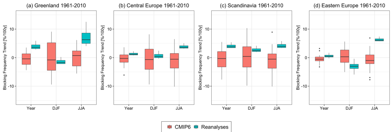
Abbildung 9: Boxplots der blocking -Trends (jährliche, winterliche und sommerliche Trends) in den Regionen. Die drei horizontalen Linien zeigen das erste und dritte Quartil, sowie den Median. Striche zeigen den Ensemble-Range, sind aber auf das 1,5-fache des Interquartilsabstands begrenzt. Trendwerte außerhalb dieses Bereichs sind durch Punkte gekennzeichnet.
