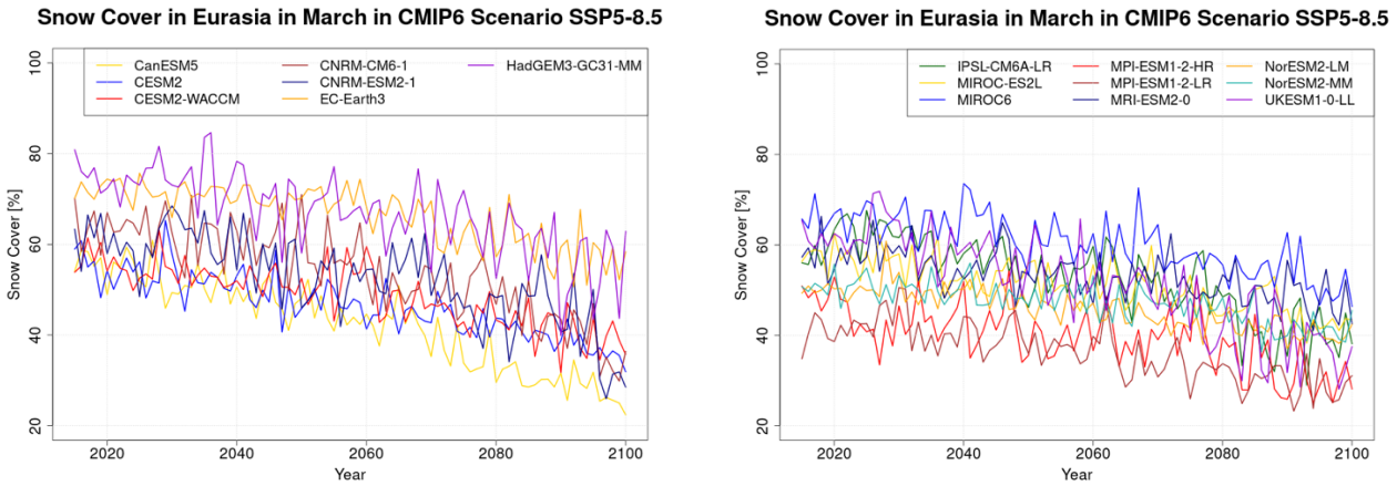
Abbildung 30: Mittlere Schneebedeckung im März über Eurasien (40°-80°N, 0°-120°O) in SSP5-8.5-Szenario. Zur besseren Übersichtlichkeit werden die Zeitserien in 2 Graphen gezeigt.
