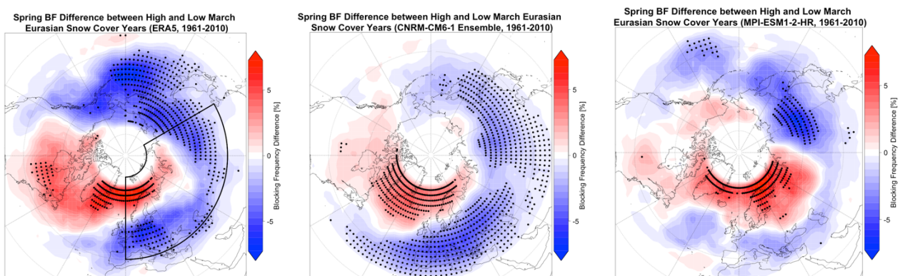
Abbildung 29: Differenz der Frühlings- blocking -Frequenz zwischen Jahren mit hoher und niedriger Schneebedeckung in Eurasien im März (1961-2010) in ERA5-Reanalyse (links), CNRM-CM6-1 (Mitte) und MPI-ESM1-2-HR (rechts). Punkte kennzeichnen Signifikanz auf dem 5%-Niveau. Die Box in der linken Abbildung kennzeichnet die Region, in der die Schneebedeckung betrachtet wird.
