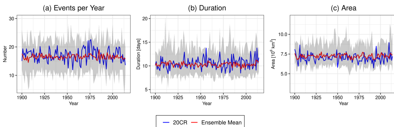
Abbildung 8: Zeitliche Entwicklung der Anzahl pro Jahr (a), der mittleren Dauer (b) und der mittleren räumlichen Ausdehnung (c) der blocking -Ereignisse für die 20CR-Reanalyse (blau), das CMIP6-
