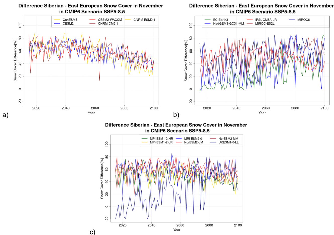
Abbildung 34: Wie in Abbildung 32 die Differenz in der mittleren Schneebedeckung, aber in CMIP6-Simulationen einer SSP5-8.5-Zukunft.
