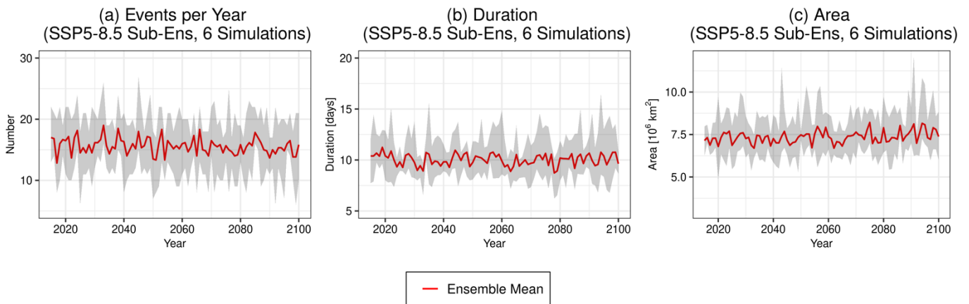
Abbildung 12: Zeitliche Entwicklung der Anzahl pro Jahr (a), der mittleren Dauer (b) und der mittleren räumlichen Ausdehnung (c) der blocking -Ereignisse für das CMIP6-Subensemblemittel (rot) im SSP5-8.5 Szenario, und die Bandbreite des Ensembles (grau). Es wurden alle blocks in der Region zwischen 45° und 75°N sowie 60°W und 60°O berücksichtigt.
