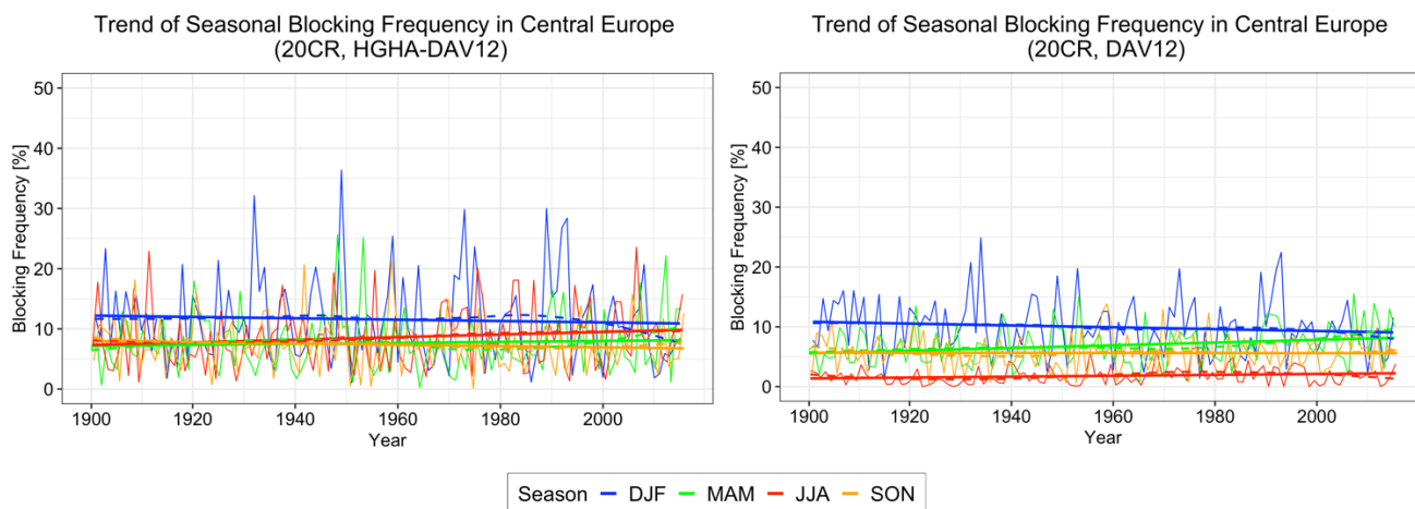
Abbildung 3: Saisonale Trends der blocking -Frequenz in Mitteleuropa (45°-60°N, 0°-20°O) auf Basis von 20CR mit HGHA-DAV12 (links) und DAV12 (rechts).
