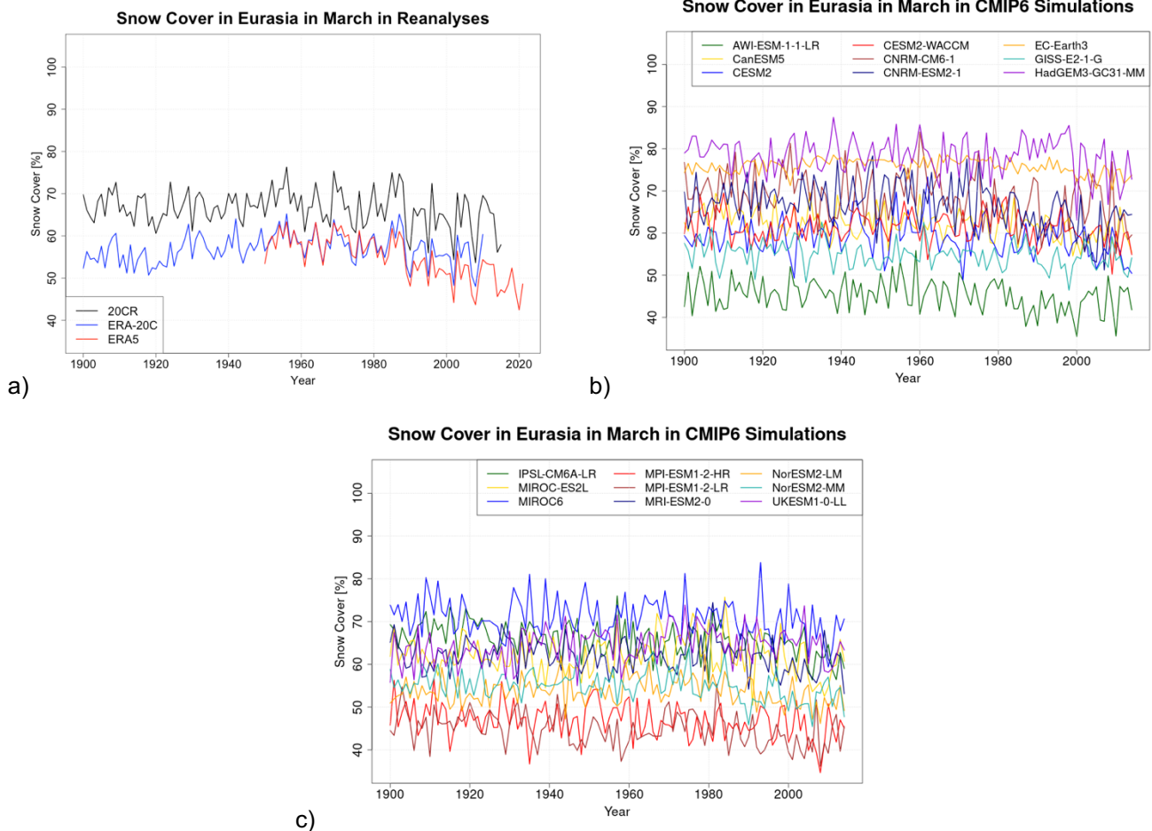
Abbildung 28: Mittlere Schneebedeckung im März über Eurasien (40°-80°N, 0°-120°O) in Reanalysen (a) und CMIP6-Simulationen (b,c). Zur besseren Übersichtlichkeit werden die Zeitserien der CMIP6-Simulationen in 2 Graphen gezeigt.
