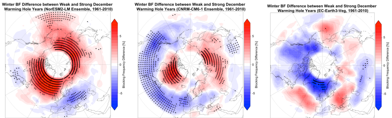
Abbildung 22: Differenz der Winter-blocking-Frequenz zwischen Jahren mit schwach und stark ausgeprägtem Erwärmungsloch im Dezember (1961-2010) in ausgewählten CMIP6-Simulationen. Punkte kennzeichnen Signifikanz auf dem 5%-Niveau.
