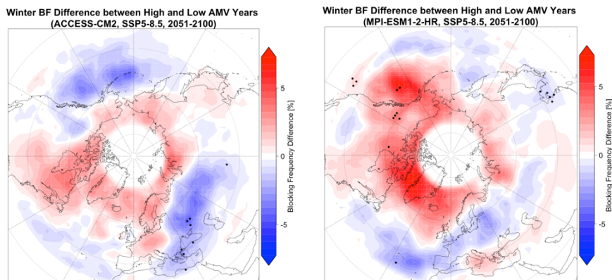
Abbildung 18: Differenz der Winter- blocking -Frequenz zwischen Jahren mit positiver und negativer AMV (2051-2100) in ACCESS-CM2 und MPI-ESM1-2-HR im SSP5-8.5-Szenario. Punkte kennzeichnen Signifikanz auf dem 5%-Niveau.
